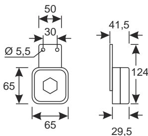
Fassung mit Anschlusskabel Bulb holder with connection cable
